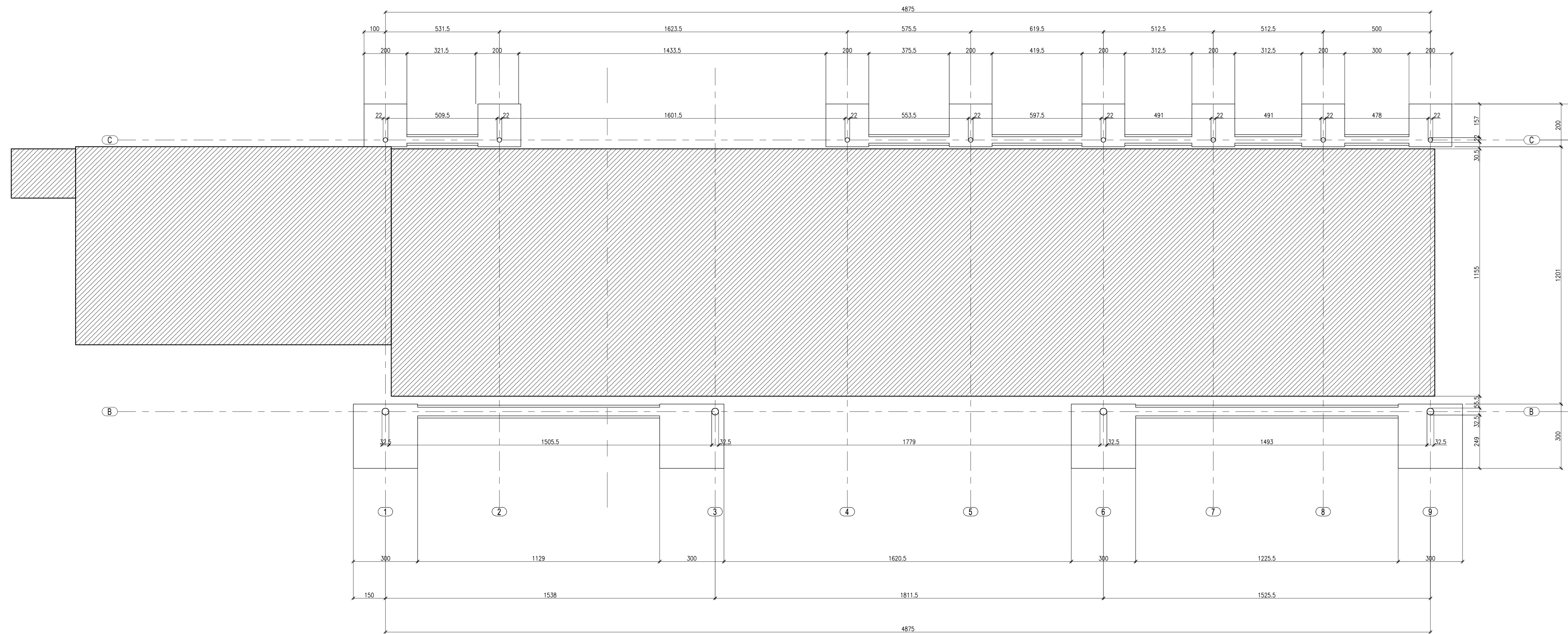
PIANTA FONDAZIONI E PILASTRI
