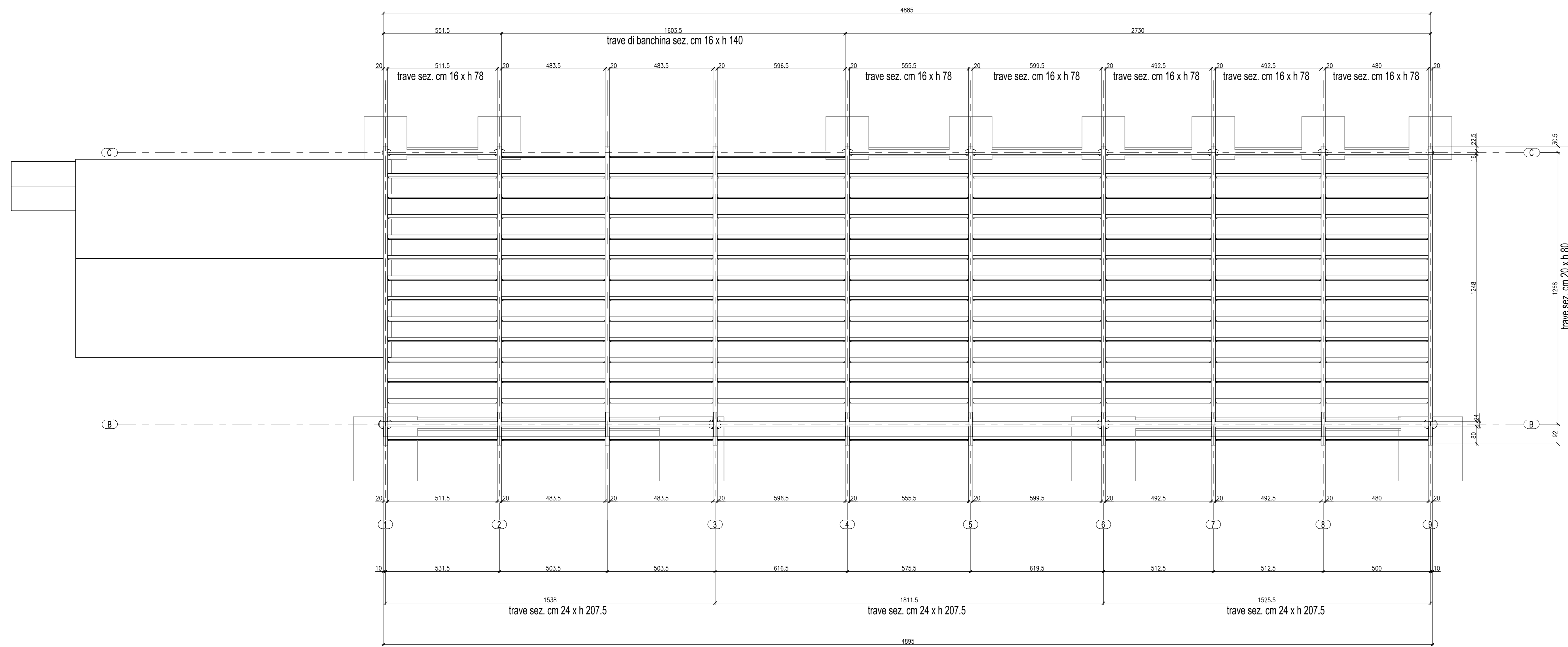
PIANTA STRUTTURE COPERTURA
